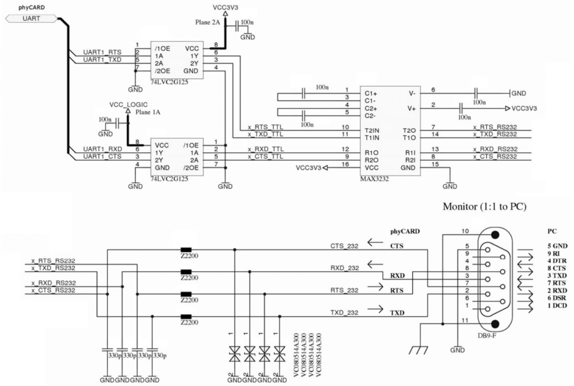
Bild 10: Beispielschaltung der UART
