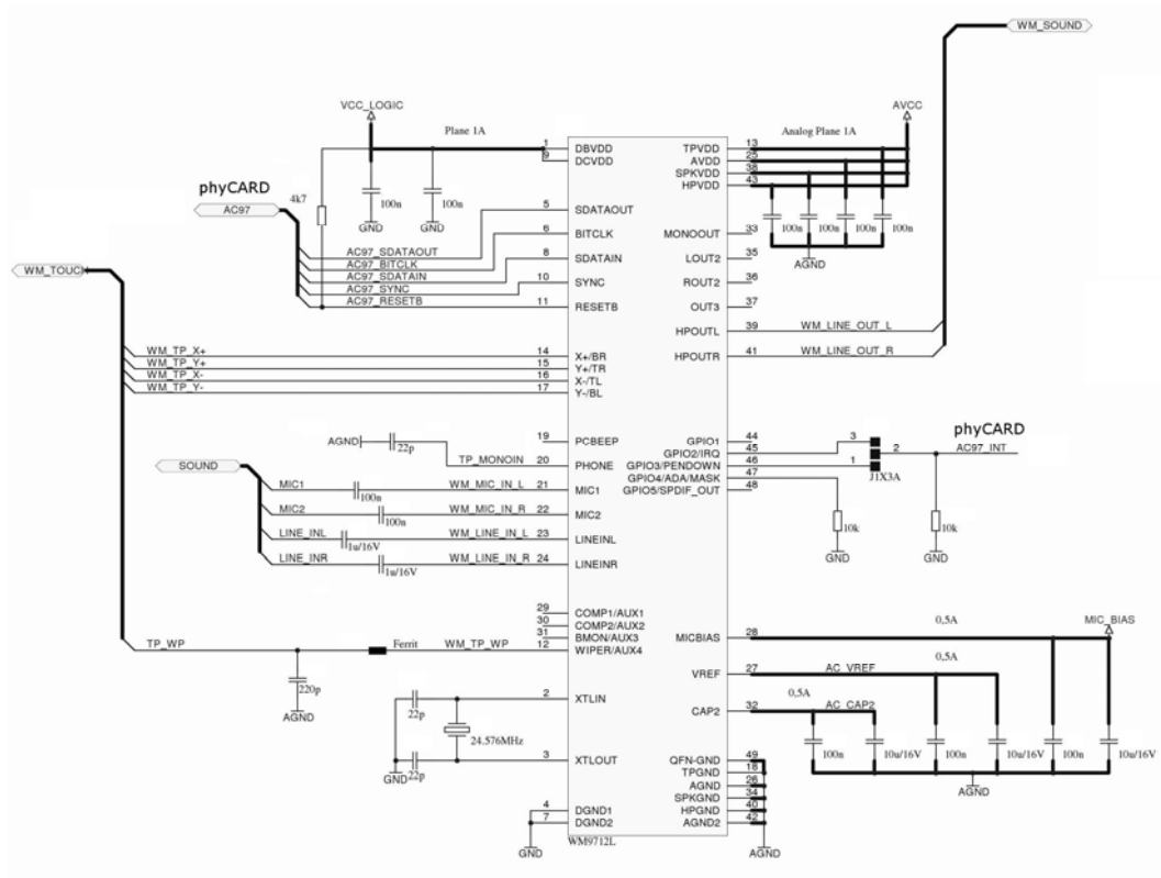
Bild 11: Beispielschaltung der AC97-Schnittstelle
