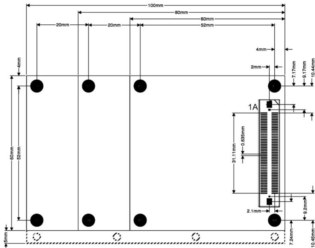
Bild 1: Maßzeichnung Basisplatte phyCARD-A
