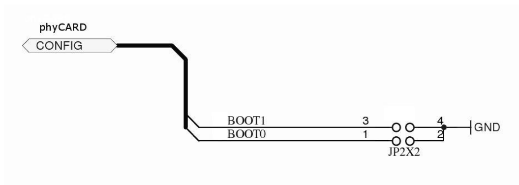
Bild 13: Beispielschaltung der Konfigurations-Pins
