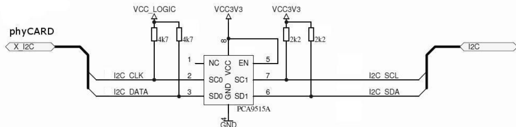
Bild 7: Beispielbeschaltung der I 2 C-Schnittstelle mit Levelshifter
