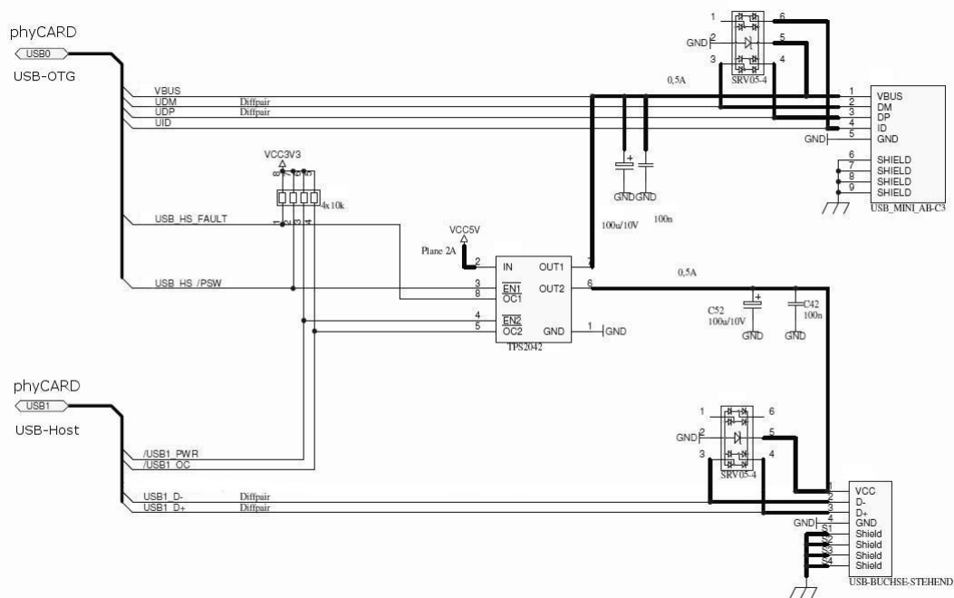
Bild 6: Beispielbeschaltung der USB-Schnittstellen
