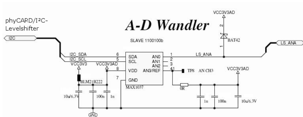
Bild 8: Beispielschaltung eines I 2 C A-D Wandlers
