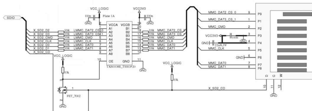
Bild 12: Beispielschaltung der SDIO-Schnittstelle
