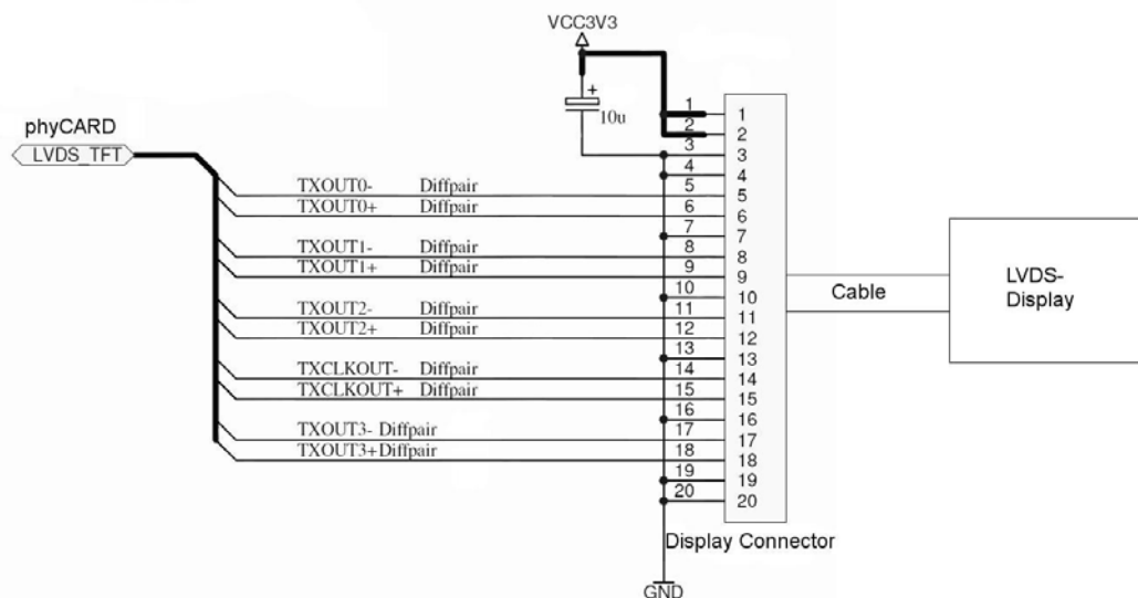
Bild 3: Beispielbeschaltung eines LVDS Display-Anschlusses
