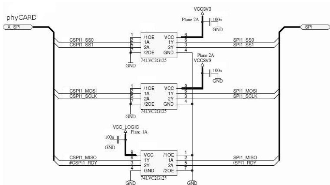
Bild 9: Beispielbeschaltung der SPI-Schnittstelle mit Levelshiftern
